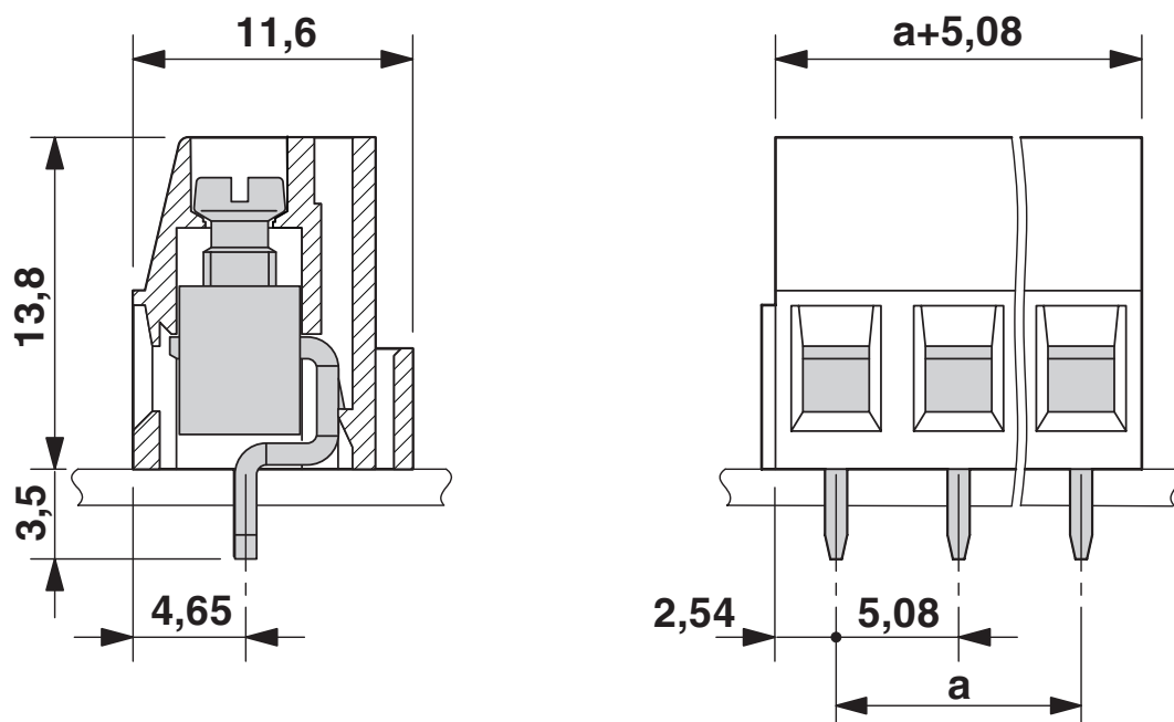
Måttskiss
