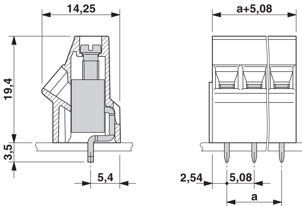
Måttskiss
