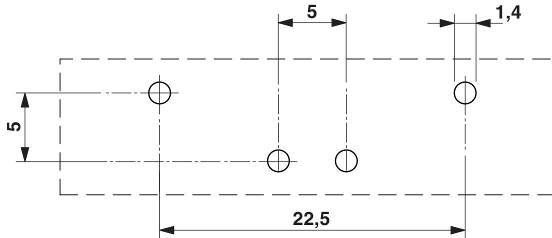
Borrplan/lödöns geometri
