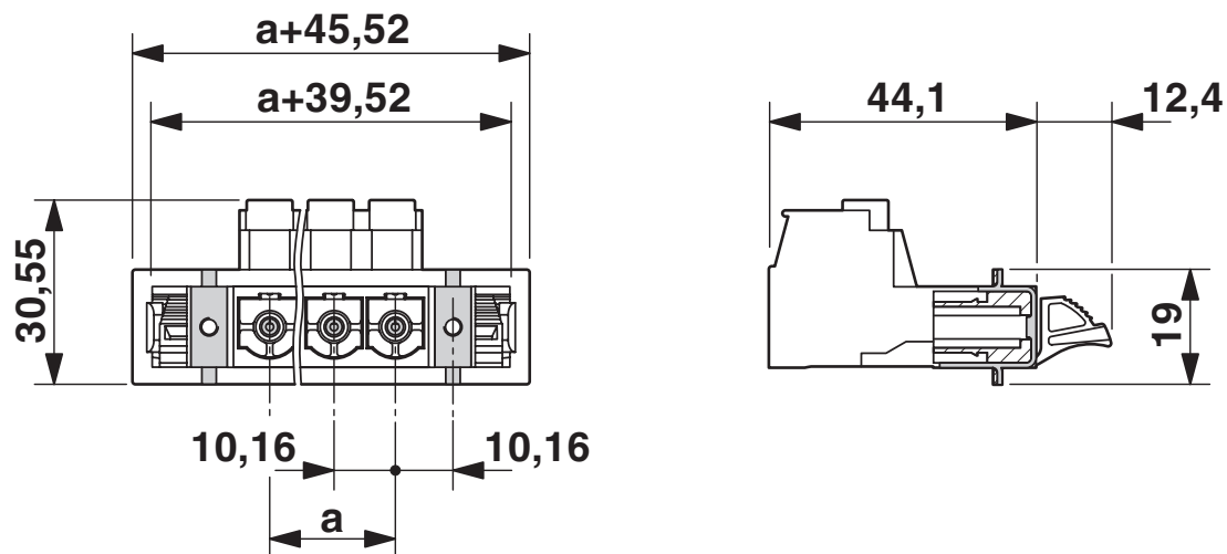
Måttskiss
