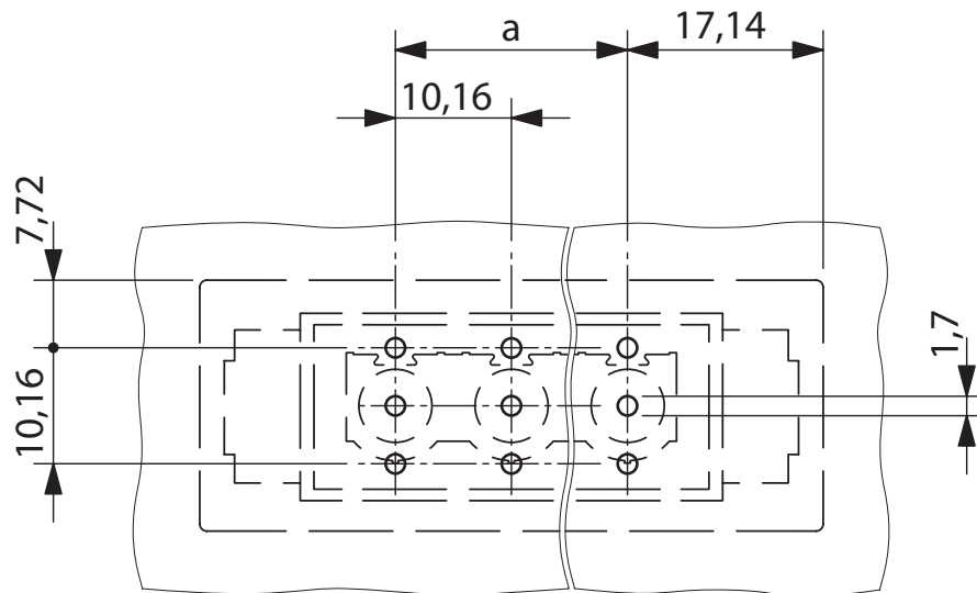
Borrplan/löddöns geometri
