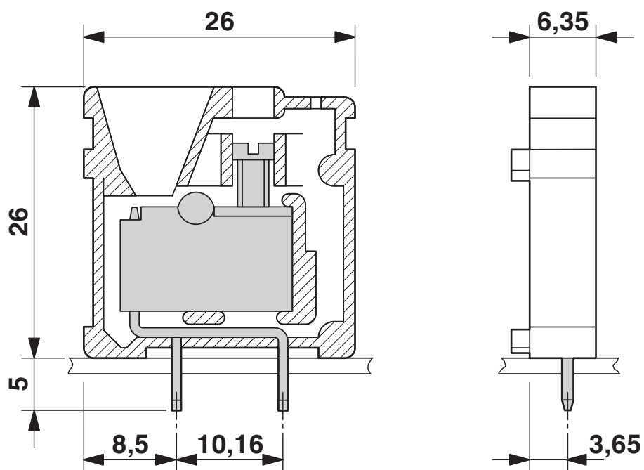
Måttskiss
