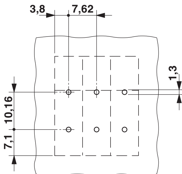
Borrplan/lödöns geometri
