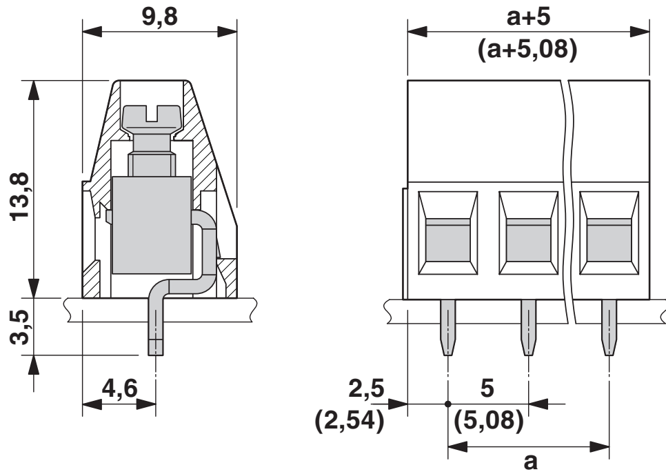
Måttskiss
