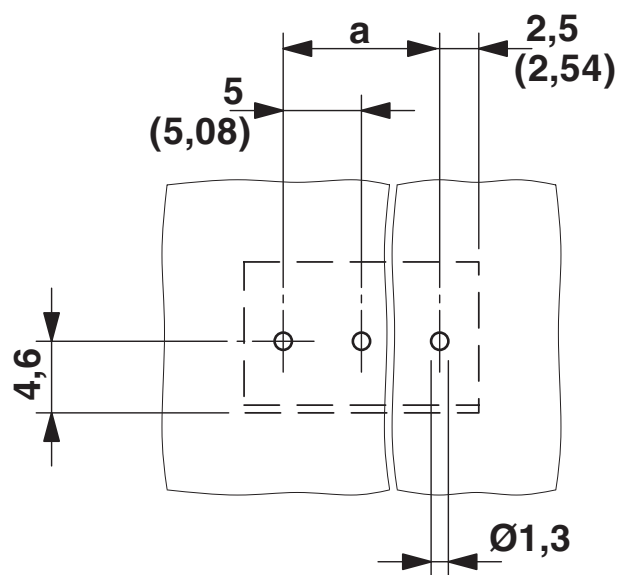
Borrplan/lödöns geometri
