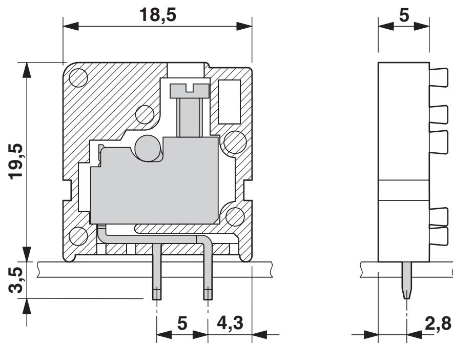
Måttskiss
