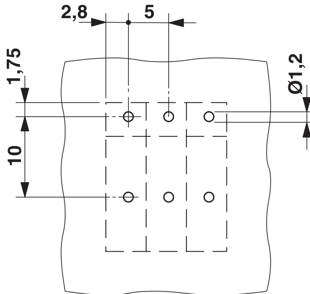
Borrplan/lödöns geometri
