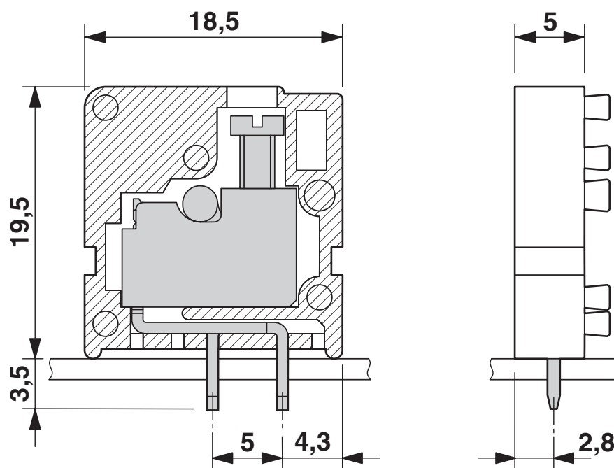
Måttskiss
