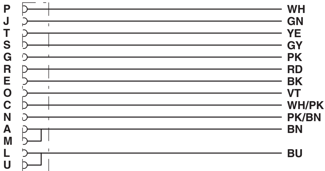
Kopplingsschema
