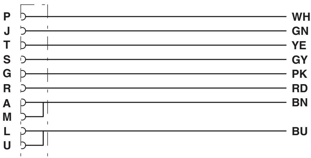
Kopplingsschema
