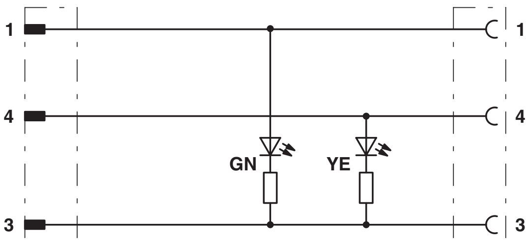
Anslutna M8-han-/honkontakter
