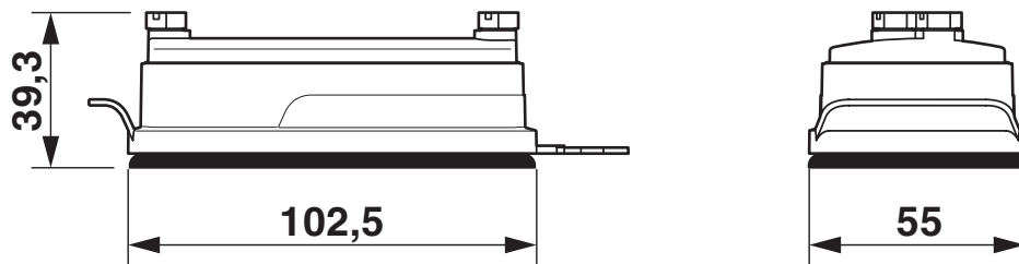
Måttskiss
