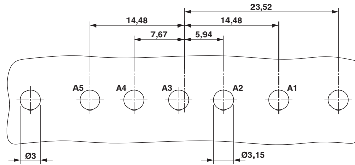
Borrplan/lödöns geometri
