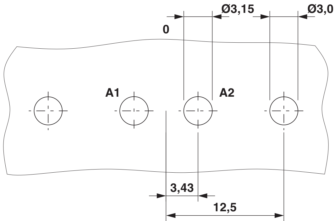
Borrplan/lödöns geometri
