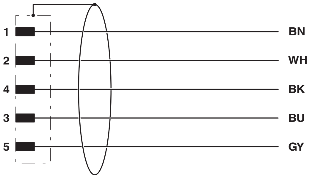
Kopplingsschema
