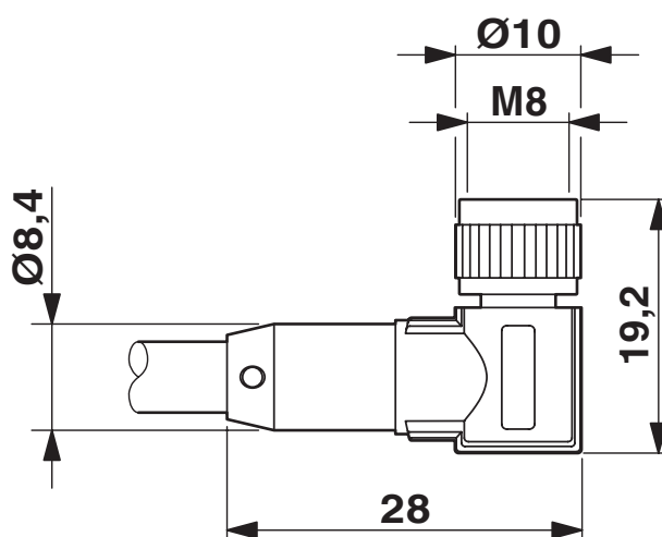
Måttskiss
