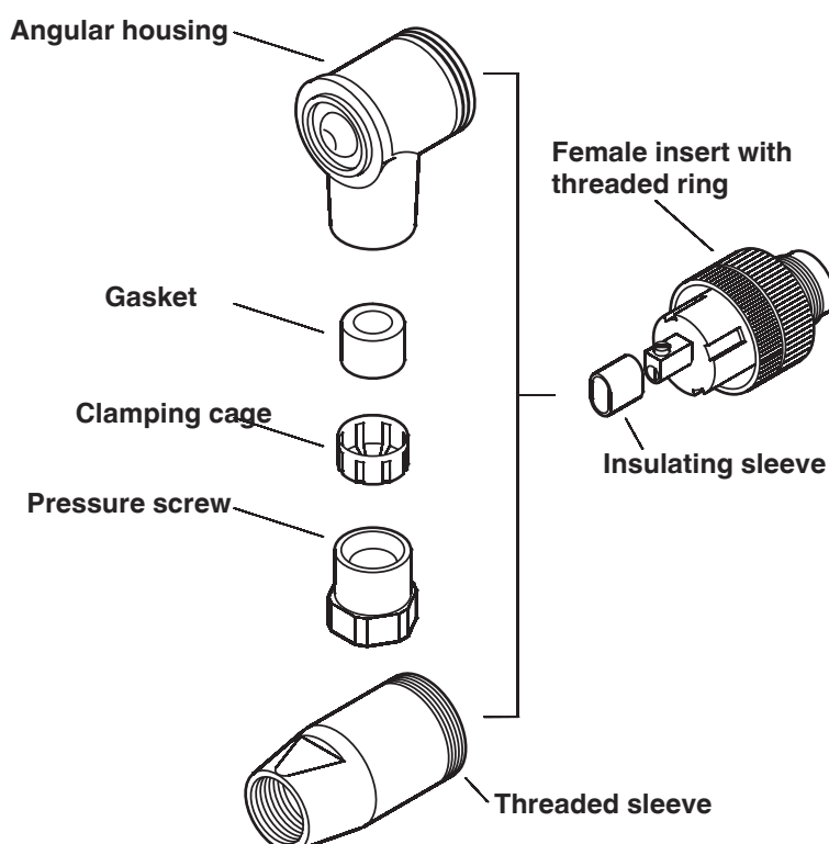
Schematisk ritning
