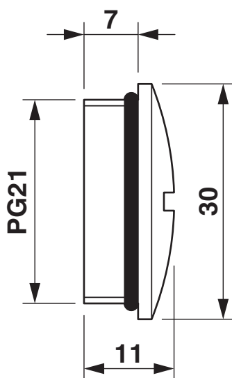
Måttskiss
