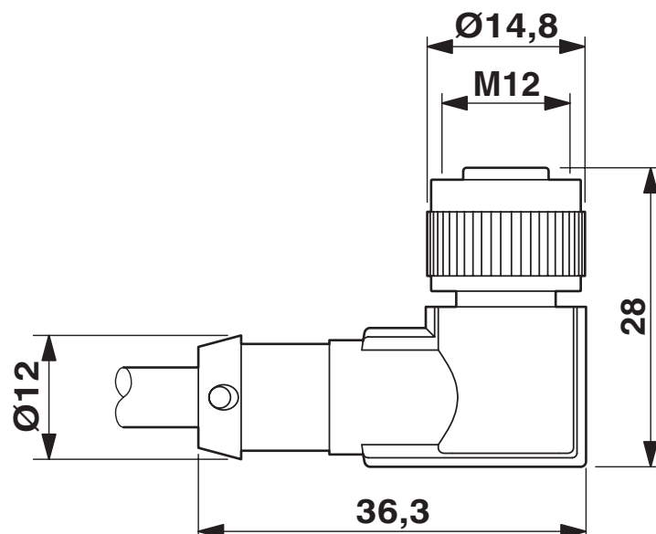
Måttskiss
