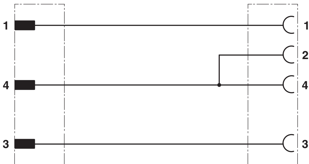
Kopplingsschema
