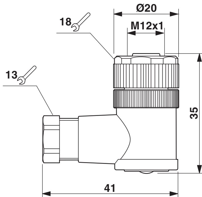
Måttskiss
