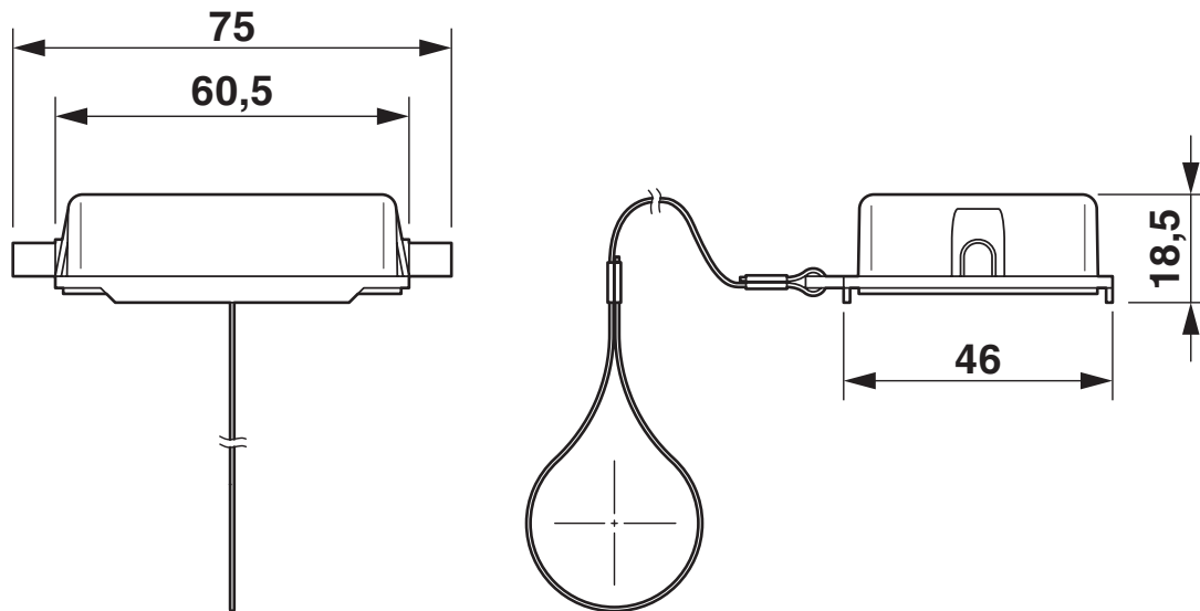
Måttskiss
