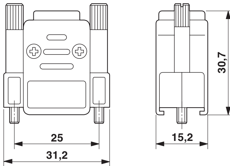
Måttskiss
