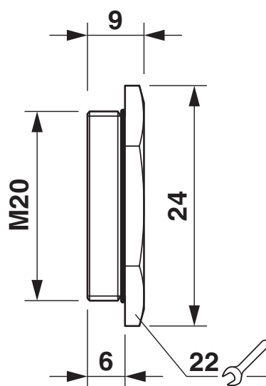
Måttskiss
