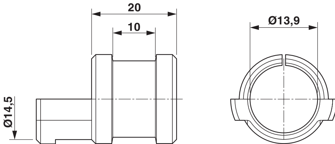
Måttskiss
