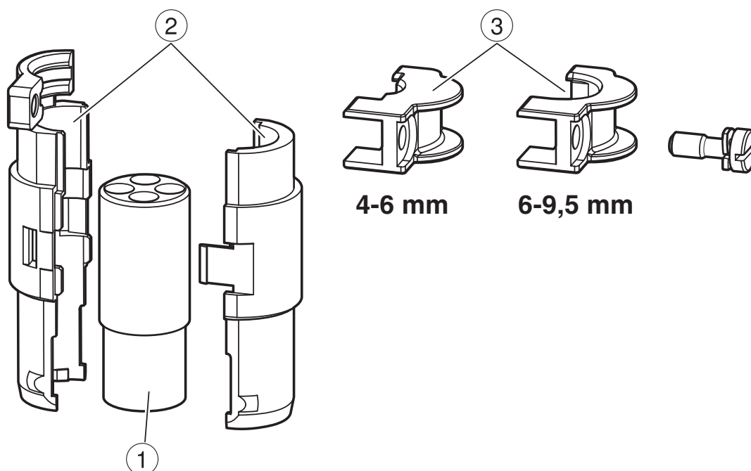
Funktionsritning
