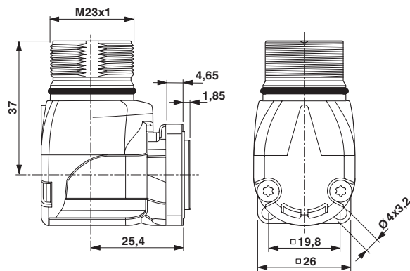
Måttskiss
