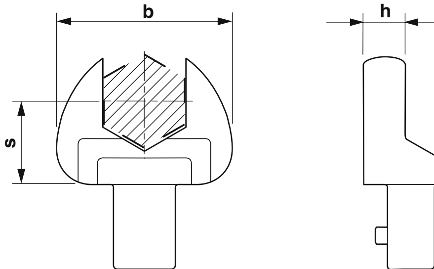
Måttskiss
