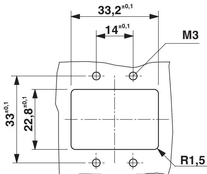
Måttskiss
