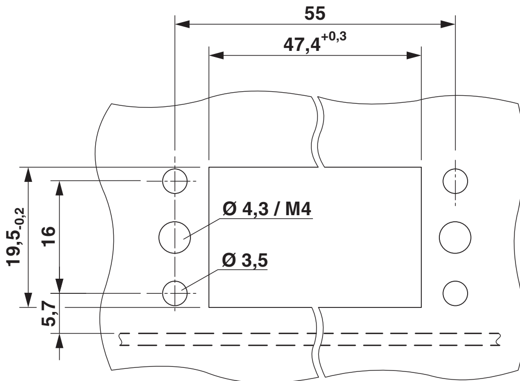
Måttskiss
