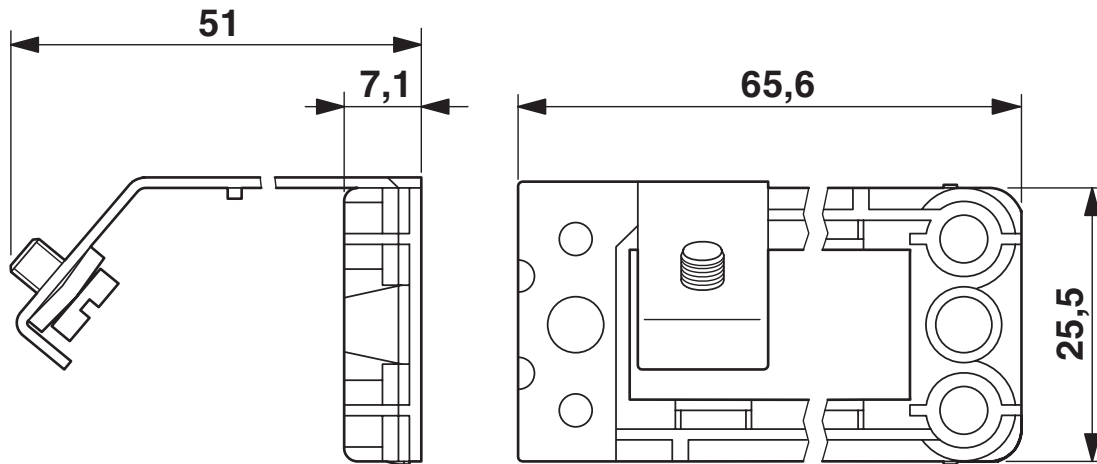
Måttskiss
