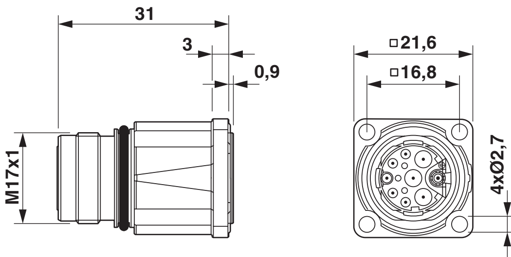
Måttskiss
