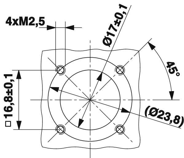
Måttskiss
