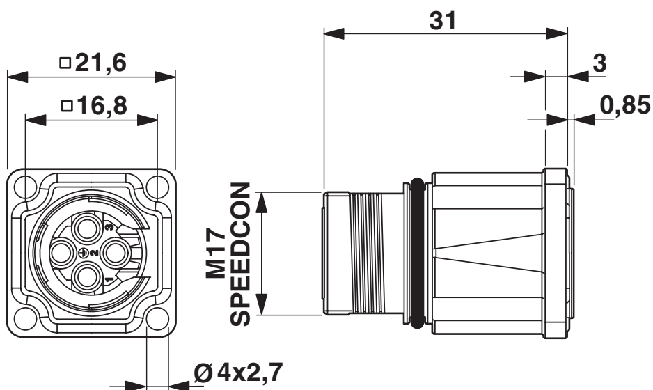
Måttskiss
