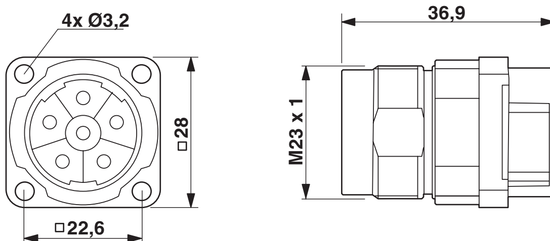
Måttskiss
