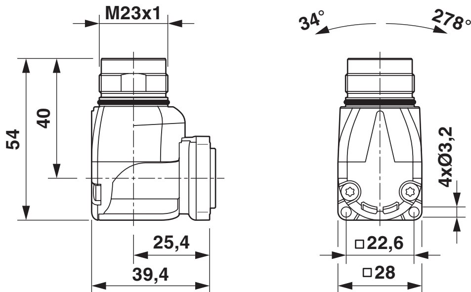
Måttskiss
