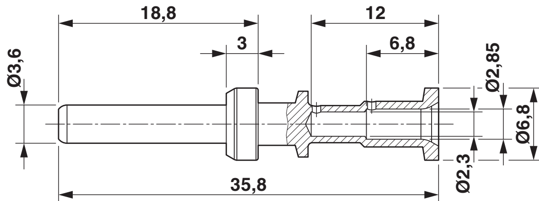
Måttskiss
