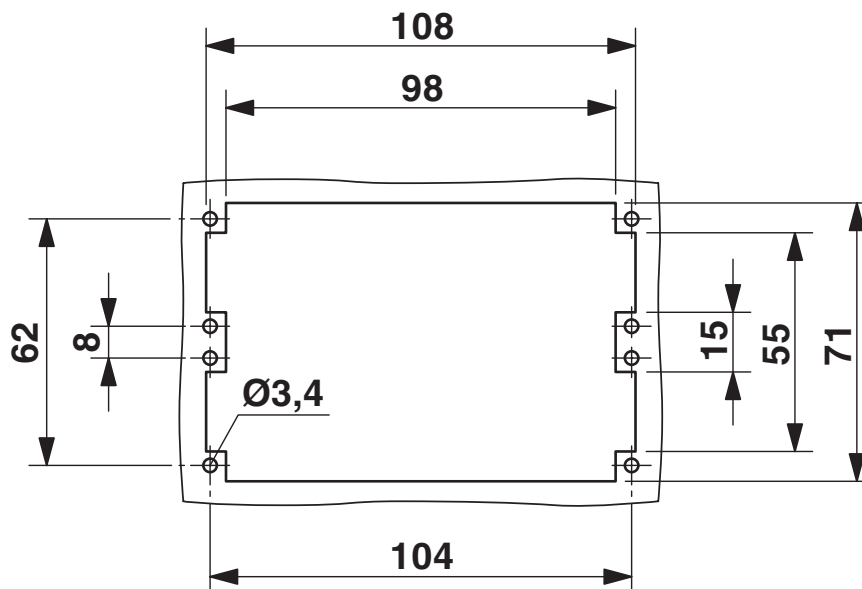
Måttskiss
