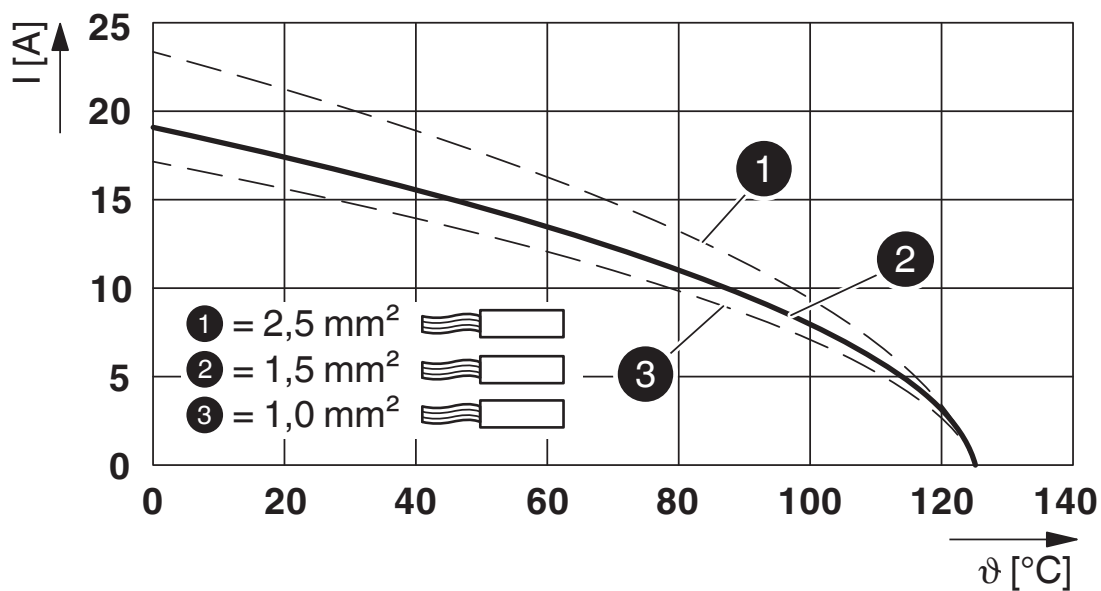
Derating-diagram för flexibel ledare
