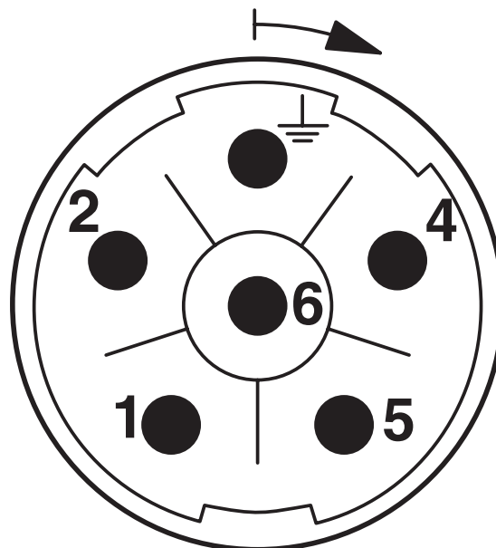
Schematisk ritning
