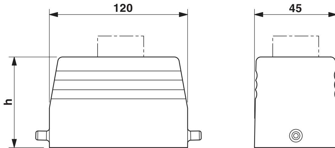
Måttskiss
