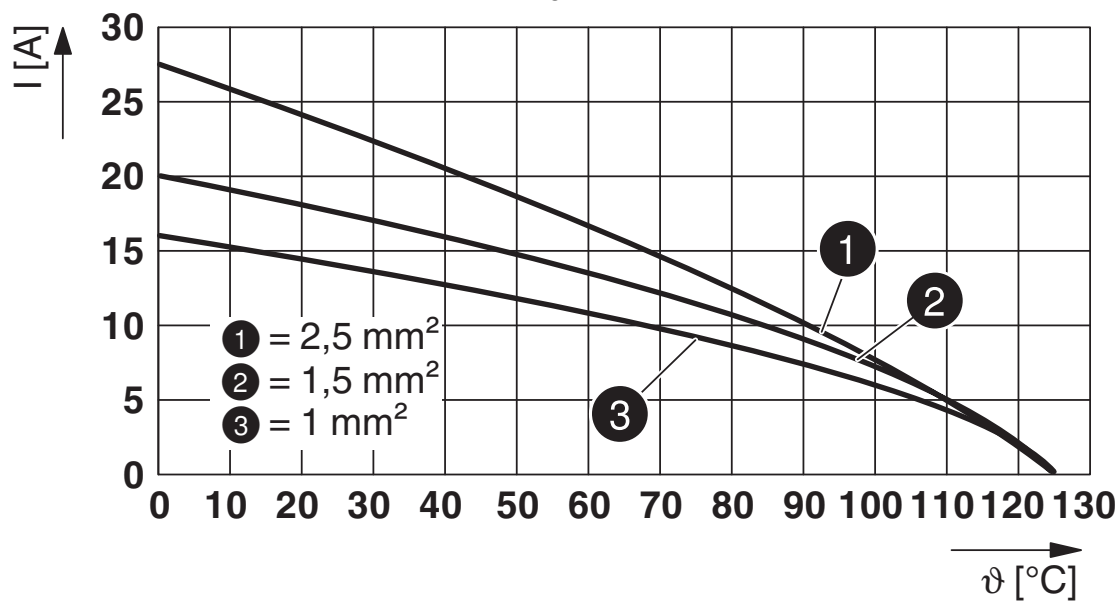
Strömbelastningskurva
