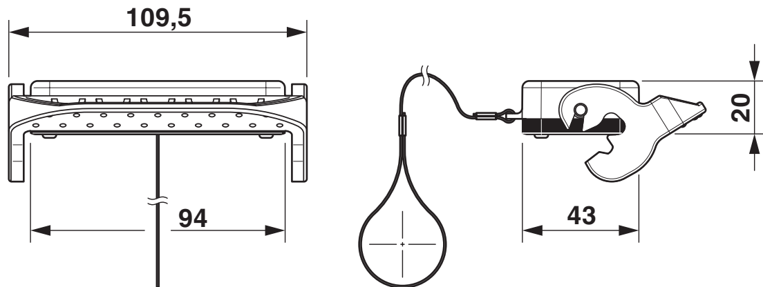
Måttskiss
