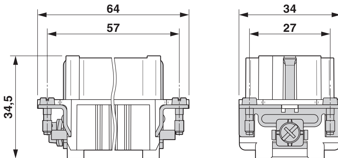
Måttskiss
