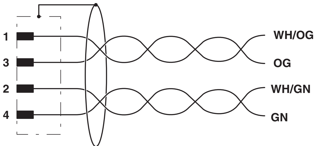
Kopplingsschema
