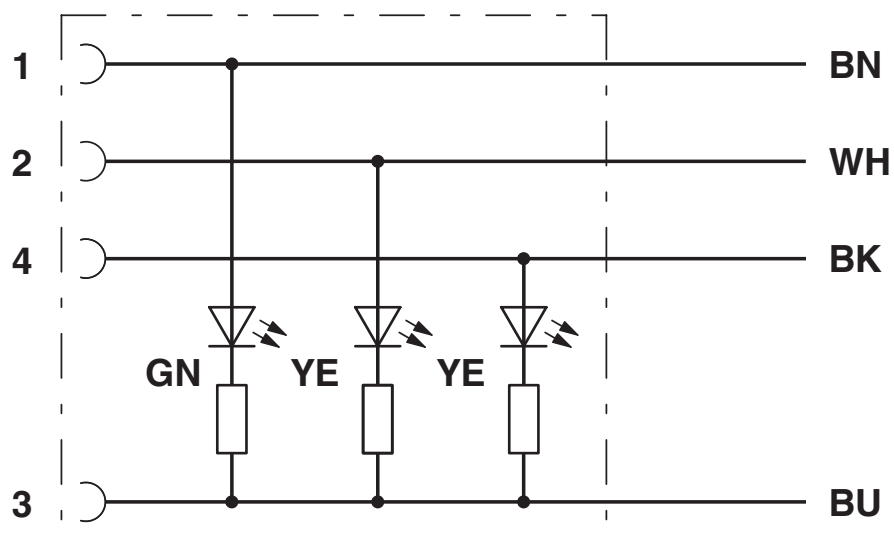
Kopplingsschema
