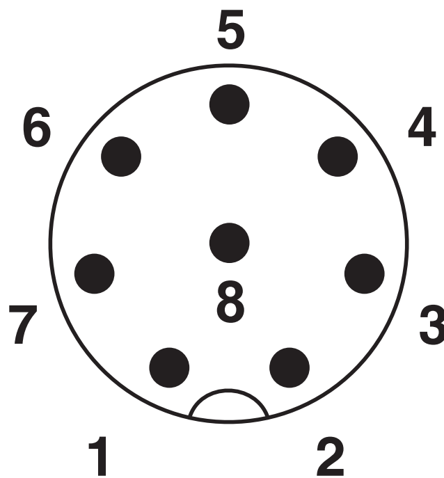
Schematisk ritning
