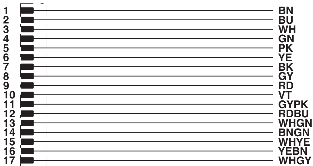
Kopplingsschema
