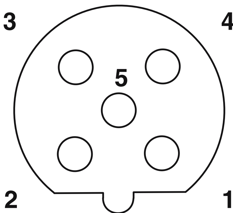
Schematisk ritning
