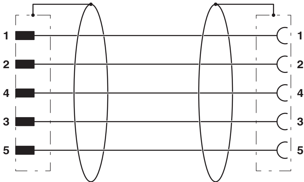
Kopplingsschema
